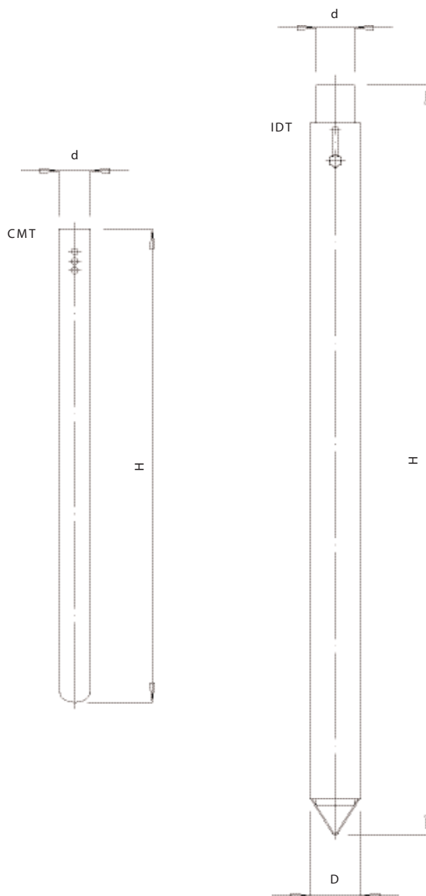
Dimensioni - Dimensions
